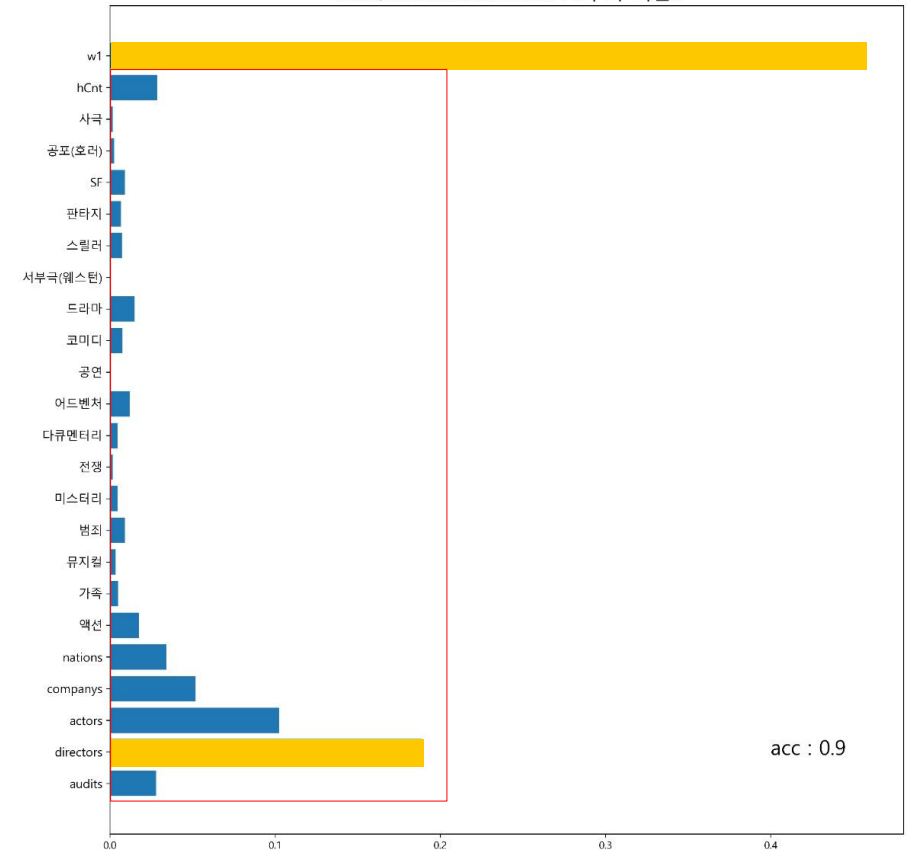
<RandomForestClassifier : 2주차 기준>
