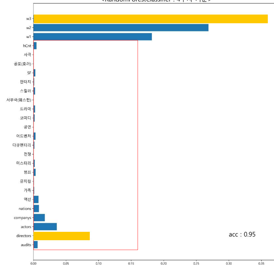
<RandomForestClassifier : 4주차 기준>
