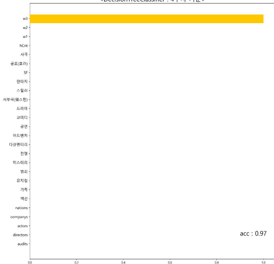
<DecisionTreeClassifier : 4주차 기준>
