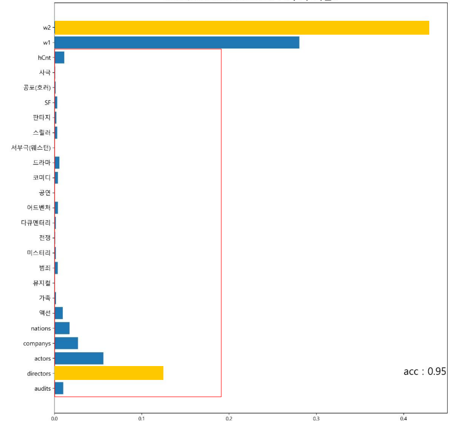
<RandomForestClassifier : 3주차 기준>
